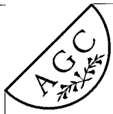
Monte Carlo
